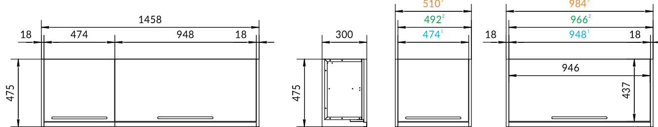
ПВ-1 Модуль с пылесосом (встраивается в верхний ящик напольной тумбы).
