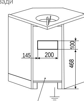
Вид модуля сзади А-10-2М
