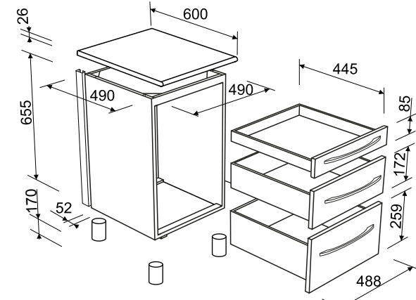
Вид модуля сзади П-10М
