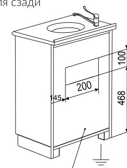
Вид модуля сзади А-10М*
