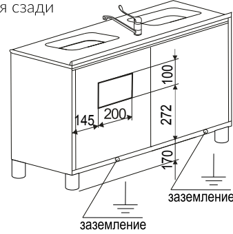
Вид модуля сзади П-10М*
