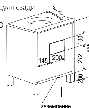
Вид модуля сзади П-10-2М
