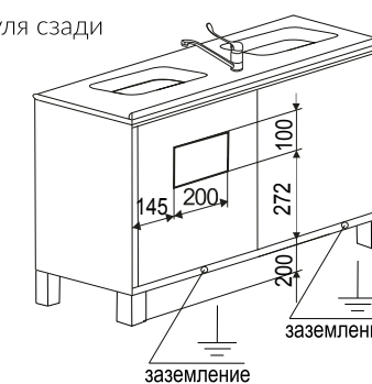
Вид модуля сзади П-10М*
