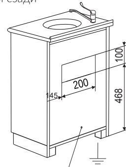
Вид модуля сзади А-10М*
