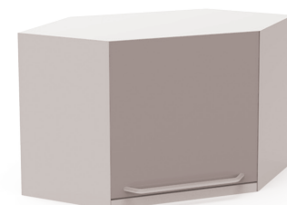
A-17U* угловой подвес- ной модуль с дверцей и полкой с кронштейном для крепления Высота: 525 мм Ширина: 683 мм Глубина: 683 мм
