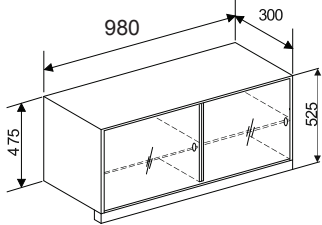
Технические характеристики: подвесные модули
