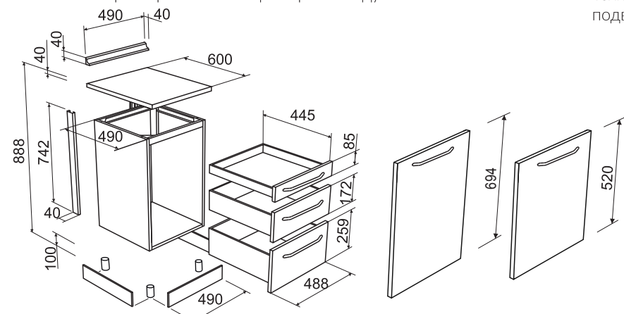
Вид модуля сзади А-10М
