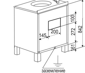
Вид модуля сзади П-10М
