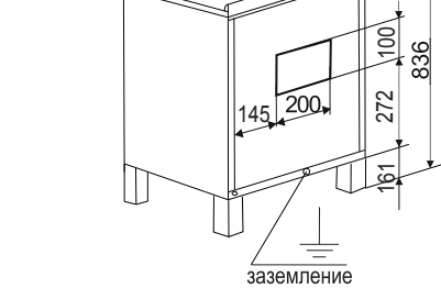
Вид модуля сзади П-10М П-10МО
