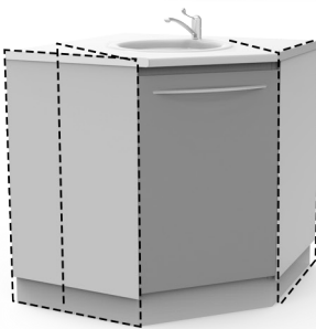
A-10M* модуль угловой с мойкой из акрила, смесителем и корзиной для мусора Высота: 876 мм Ширина:910 мм Глубина: 910 мм
