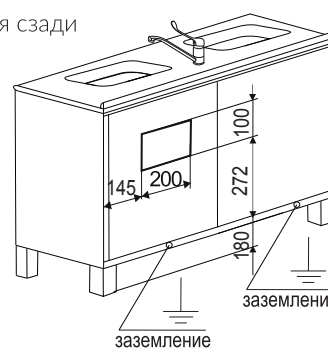
Вид модуля сзади П-10М*
