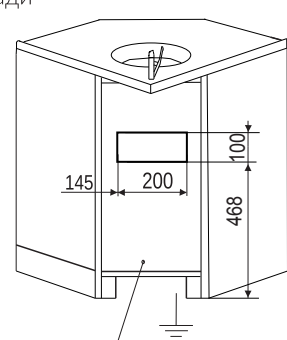
Вид модуля сзади А-10-2М
