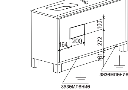
Вид модуля сзади П-10-2М
