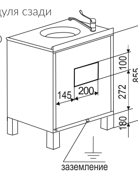
Вид модуля сзади П-10-2М
