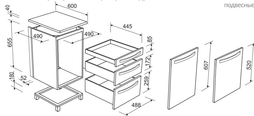
Вид модуля сзади П-10М П-10МО
