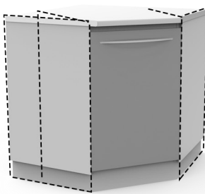
A-10* модуль угловой с дверцей и 2 полками Высота: 876 мм Ширина:910 мм Глубина: 910 мм
