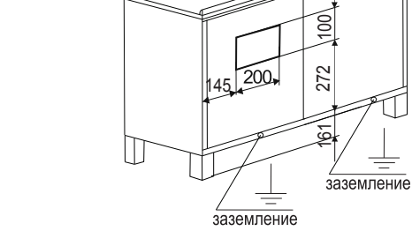
Вид модуля сзади П-10-2М
