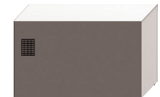
Ш-2 модуль шумоизоляци- онный на компрессор с дверью и вентиля- тором Высота: 700 мм Ширина: 1200 мм Глубина: 600 мм
