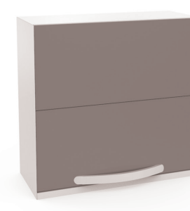
А-16Д подвесной модуль с нижней подсветкой с дверцей и 1 полкой Высота: 785 мм Ширина: 784 мм Глубина: 336 мм
