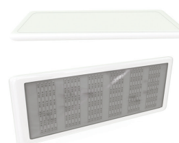
3-03, 3-04 - (нерж.) зонт с вытяжным устройством и подсветкой Высота: 635 мм Ширина: 1080 мм Глубина: 600 мм 25600 р. 35300 р.
