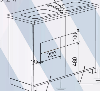
Вид модуля сзади А-10-2М
