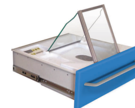
БН-1 подвесной модуль гигиенический Высота: 270 мм Ширина: 380 мм Глубина: 112 мм
