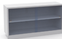
A-16 модуль настенный подвесной с раздвижными стеклянными дверцами, полкой и нижней подсветкой Высота: 525 мм Ширина: 1100 мм Глубина: 400 мм
