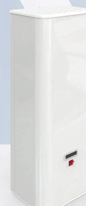
A-05Б (на 4 лампы) рециркуля- тор воздуха (вертикальный, горизонтальный) с кнопкой вклю- чения и дисплеем Высота: 655 мм Ширина: 175 мм Глубина: 130 мм
