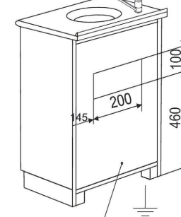
Вид модуля сзади А-10М
