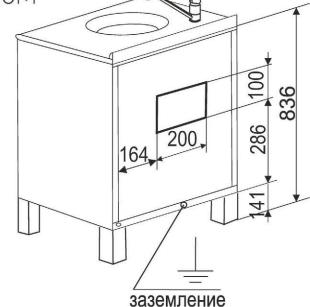
Вид модуля сзади П-10М
