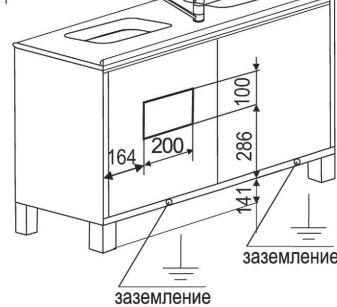
Вид модуля сзади П-10-2М
