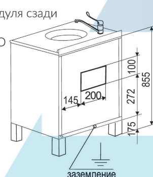
Вид модуля сзади П-10М П-10МО
